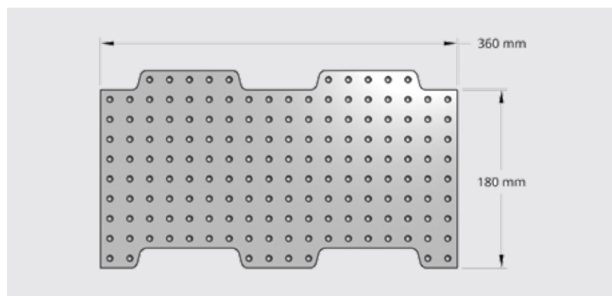
Palette 360×180 Pallet 360×180
