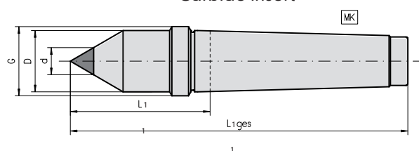
Type 507 DIN 807 HE Hartmetalleinsatz mit halber Spitze Carbide insert with half cone point
