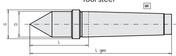
Type 505 DIN 807 WS Werkzeugstahl Tool steel
